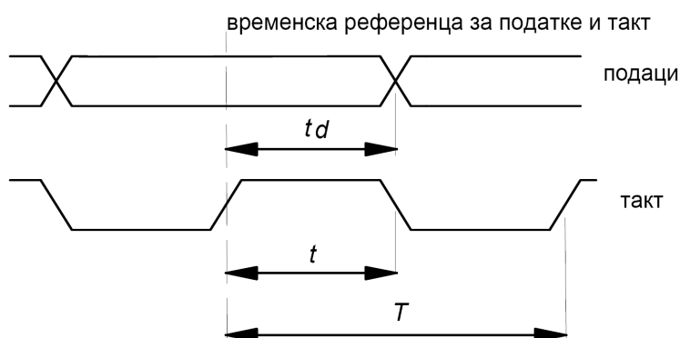
Слика 9 - Такт у односу на сигнал података
