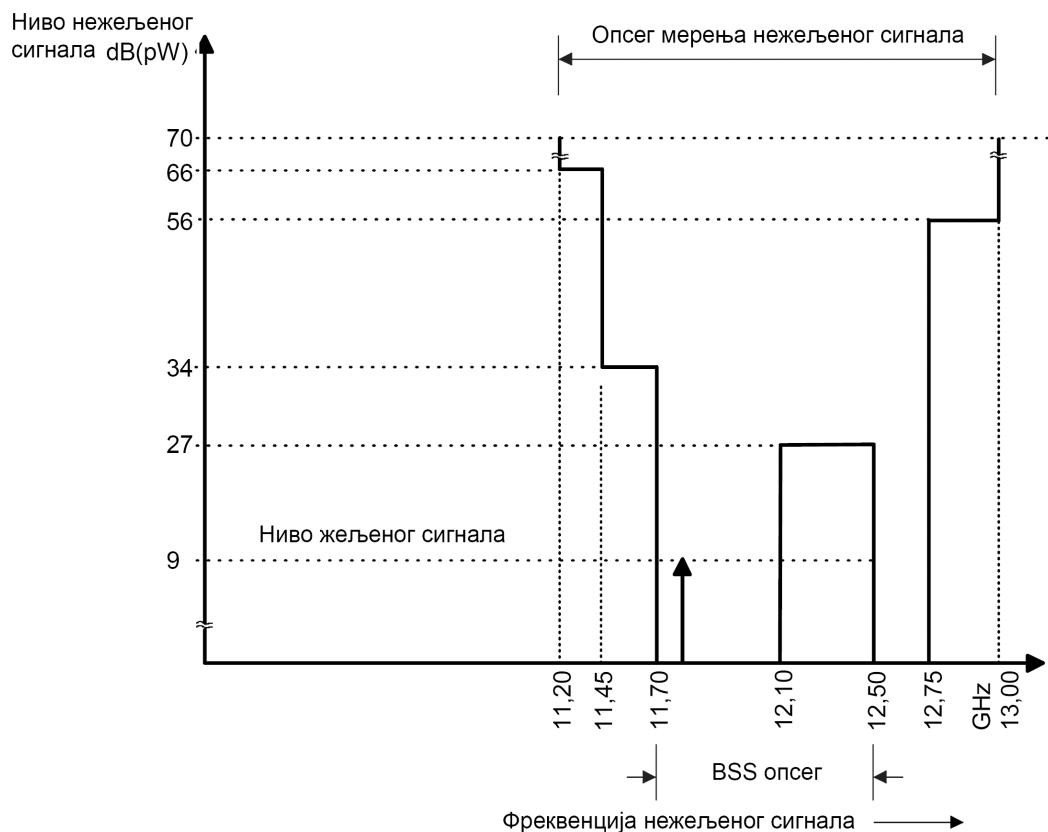
Слика 6 - Нивои жељених и нежељених сигнала интерне имуности BSS спољних јединица
