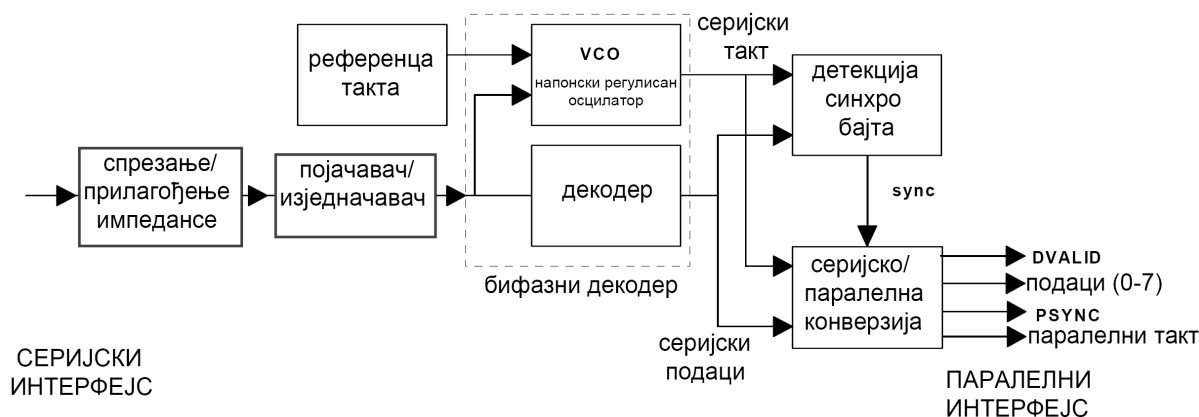
Слика Ц.3 - Пример имплементације пријемног модула
