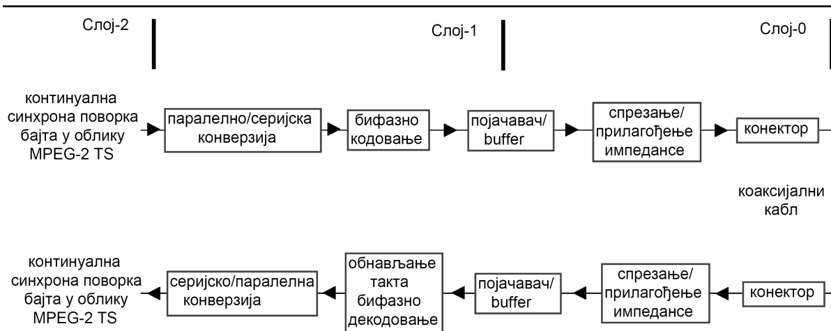
Слика А.2 - Синхрони серијски вод преноса (SSI) коаксијалним каблом
