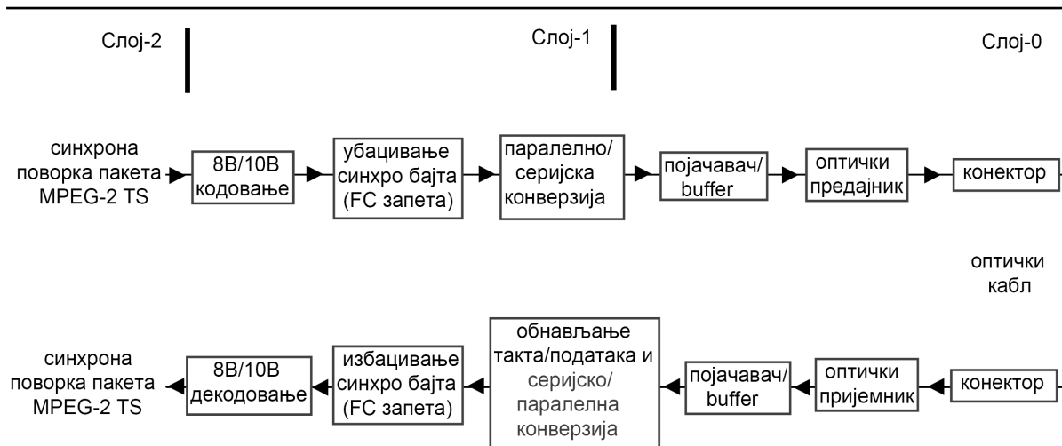
Слика Б.2: Асинхрони серијски вод преноса (ASI) оптичким каблом
