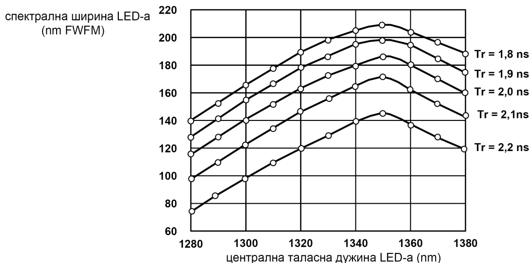
Слика Б.6 - Спектрална ширина предајника
